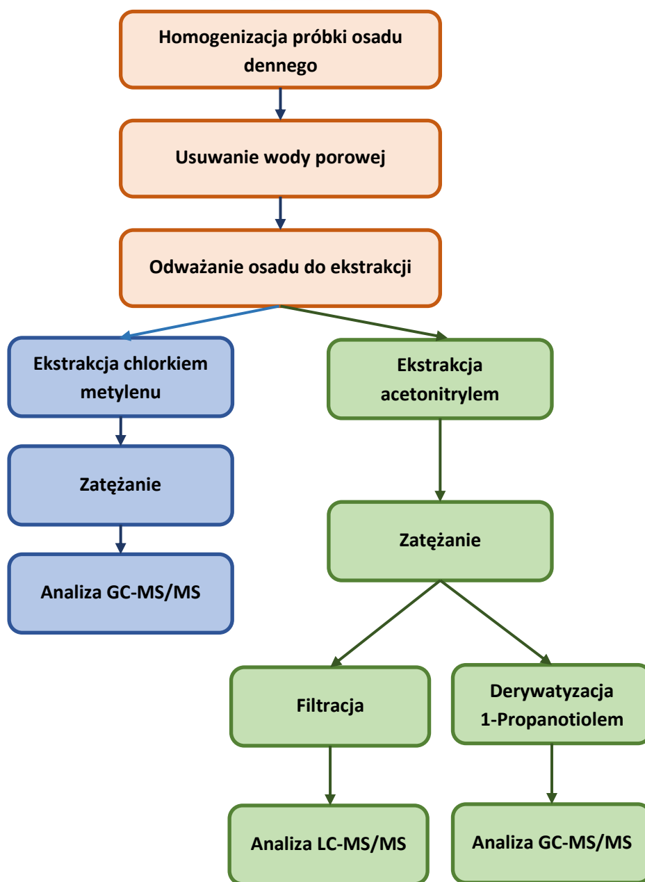
Rysunek 30. Schemat przygotowania próbek do analizy chromatograficznej (źródło: Badania 2025–2026)
