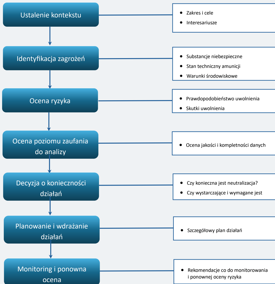
Rysunek 25. Schemat procesu zarządzania ryzykiem w odniesieniu do amunicji (źródło: opracowanie własne)
