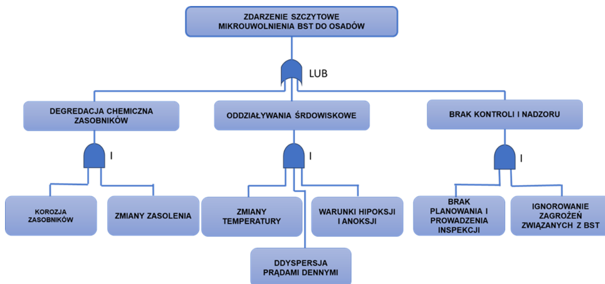
Rysunek 17. Diagram FTA dla Scenariusza 3 (źródło: opracowanie własne)
