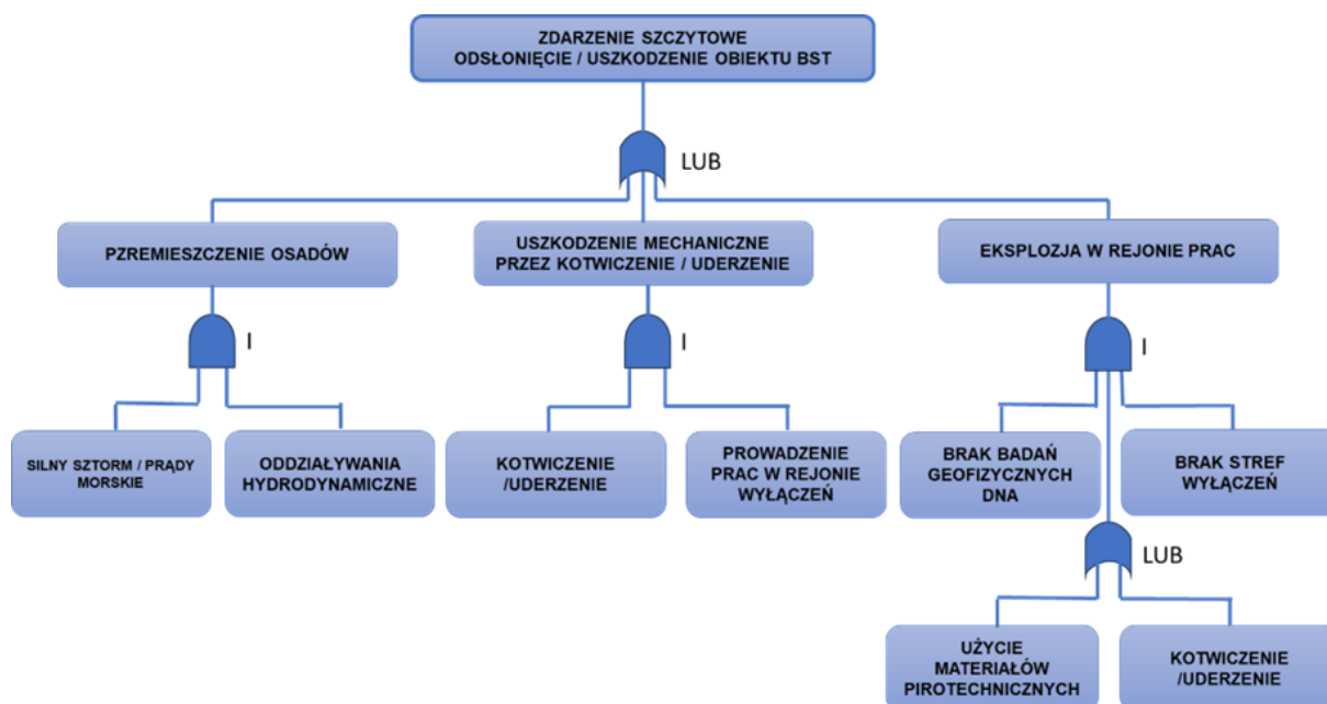
Rysunek 19. Diagram FTA dla Scenariusza 4 (źródło: opracowanie własne)
