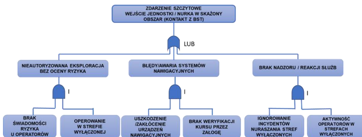
Rysunek 23. Diagram FTA dla Scenariusza 6 (źródło: opracowanie własne)
