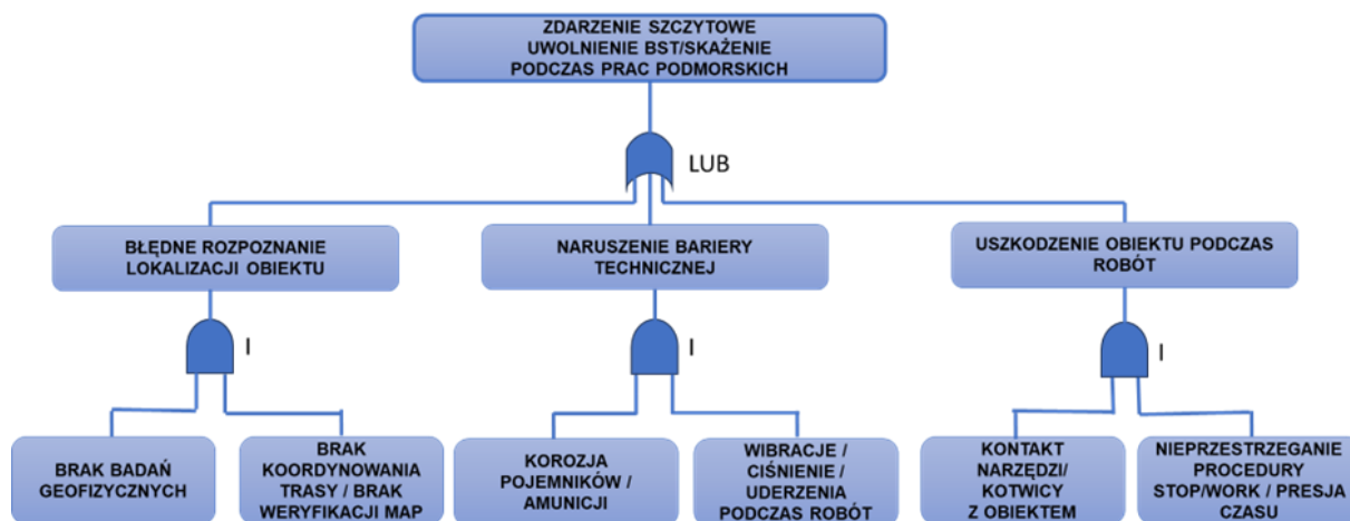
Rysunek 13. Diagram FTA dla Scenariusza 1 (źródło: opracowanie własne)
