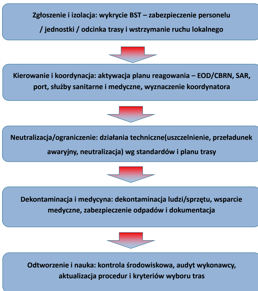
Rysunek 12. Algorytm działania dla incydentu objętego wysokim priorytetem – Scenariusz 1. Prace podmorskie (źródło: opracowanie własne)
