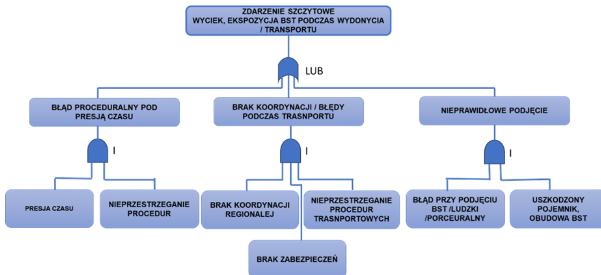
Rysunek 21. Diagram FTA dla Scenariusza 5 (źródło: opracowanie własne)
