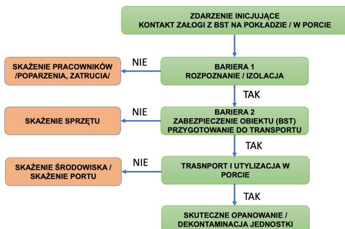
Rysunek 16. Diagram ETA dla Scenariusza 2 (źródło: opracowanie własne)
