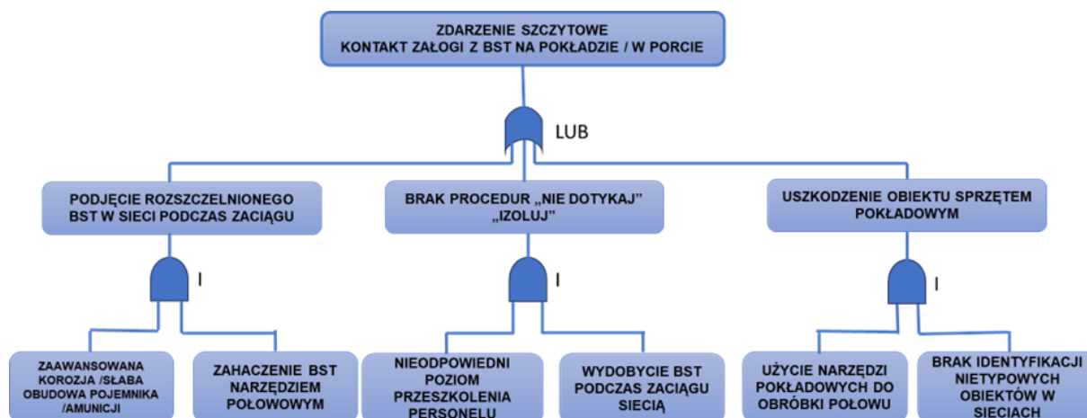
Rysunek 15. Diagram FTA dla Scenariusza 2 (źródło: opracowanie własne)
