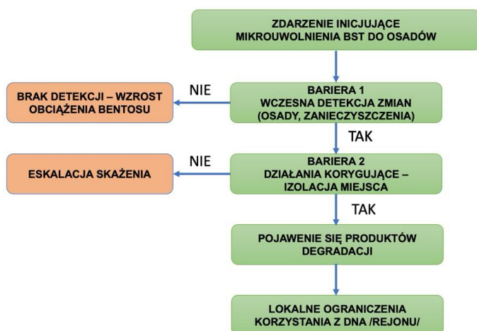
Rysunek 18. Diagram ETA dla Scenariusza 3 (źródło: opracowanie własne)
