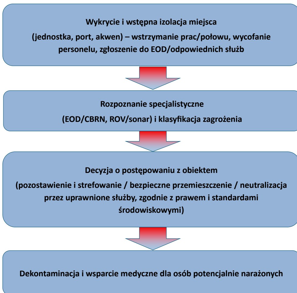
Rysunek 11. Algorytm działania dla incydentu objętego wysokim priorytetem – Scenariusz 2. Połowy denne i zaciągnięcia (źródło: opracowanie własne)
