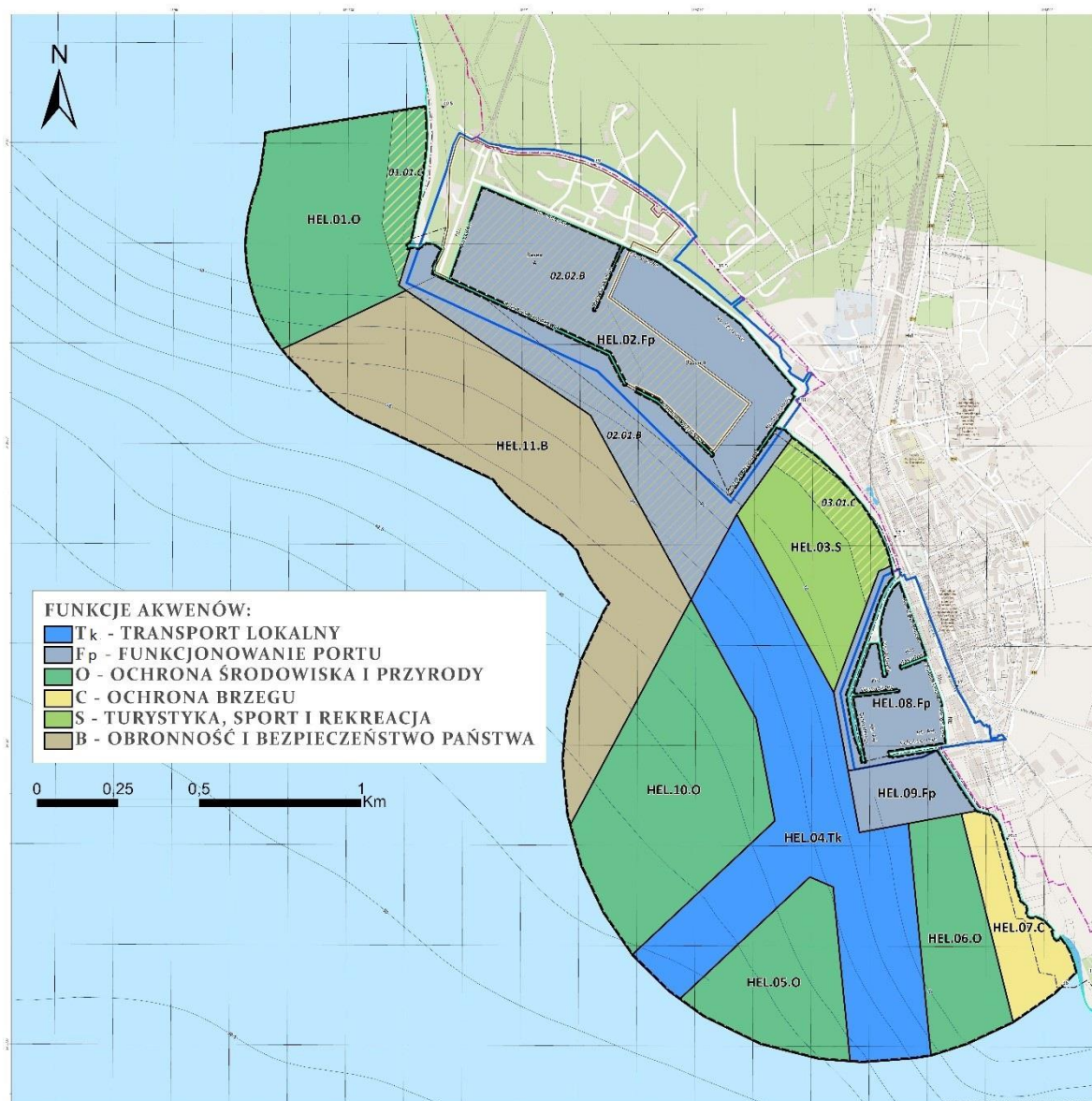
Ryc. 53. Schemat przedstawiający rysunek planu zagospodarowania przestrzennego akwenów portu morskiego w Helu – wersja v.3, funkcje podstawowe akwenów
