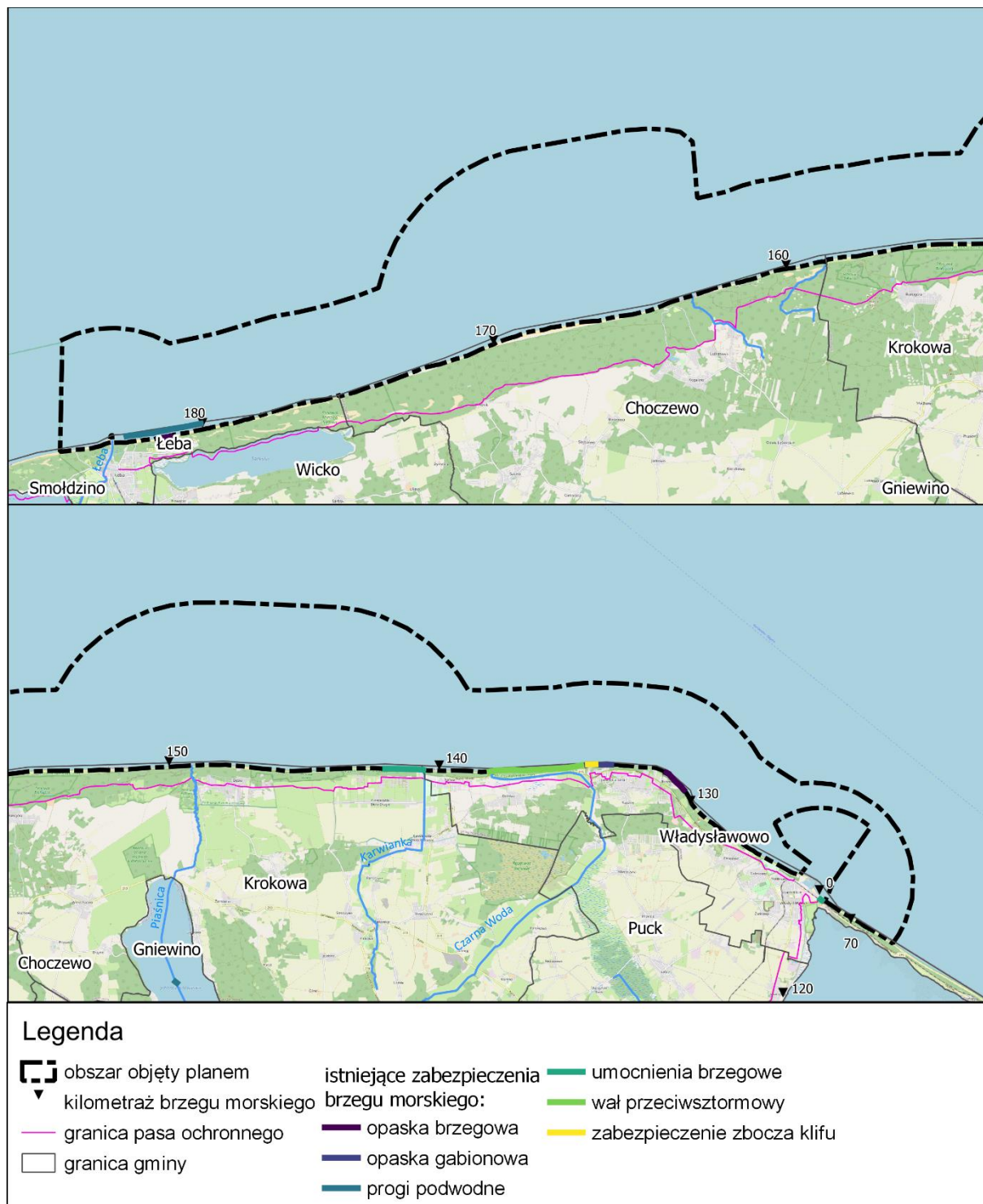
Ryc. 13. Istniejące budowle ochrony brzegu morskiego
