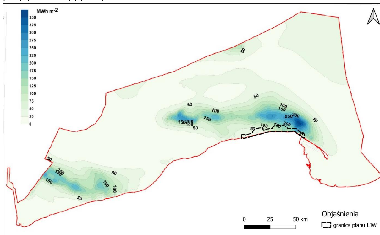
Ryc. 17. Zasoby energii przepływu wody w toni w polskich obszarach morskich obliczone dla roku 2015
