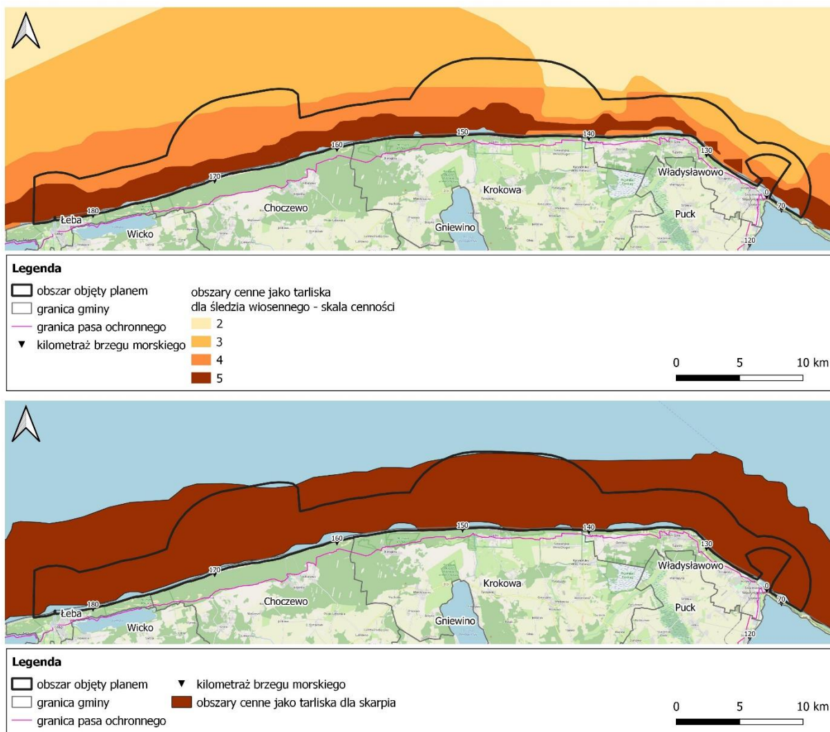
Ryc. 31. Obszary cenne jako tarliska: śledzia jesiennego (górze), śledzia wiosennego (środek) i skarpia (dół)
