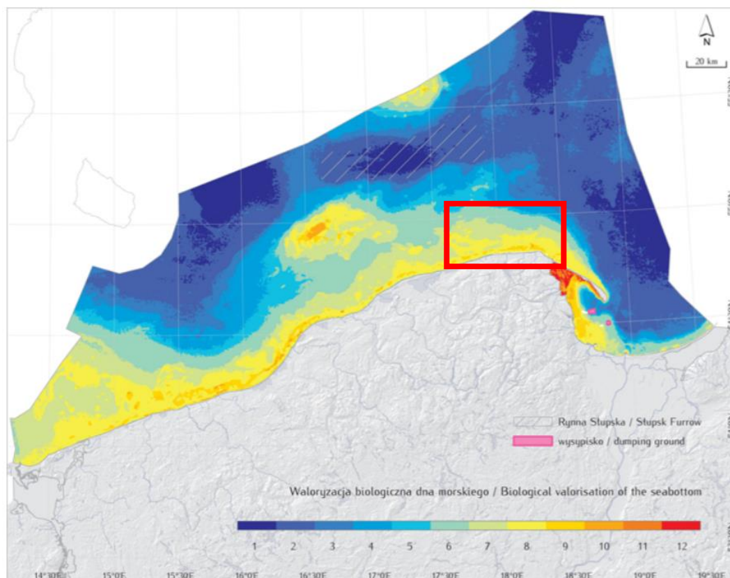
Ryc. 55. Waloryzacja biologiczna dna morskiego polskich obszarów morskich (Źródło: Atlas siedlisk polskich obszarów morskich, 2009) 108
