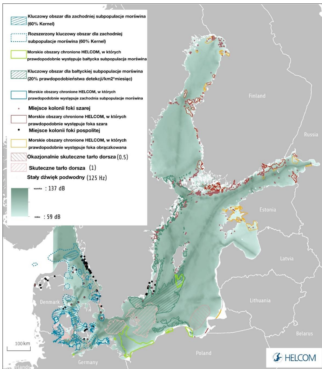
Ryc. 65. Poziom ciśnienia akustycznego (dB re 1 uPa) dla pasma 125 Hz na tle obszarów ważnych dla ssaków morskich w Bałtyku.
