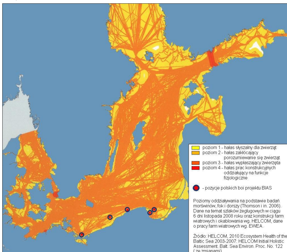
Ryc. 23. Natężenie hałasu wzdłuż szlaków żeglugowych w latach 2003 – 2007.
