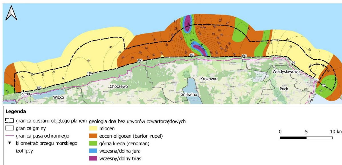
Ryc. 3. Geologia dna morskiego
