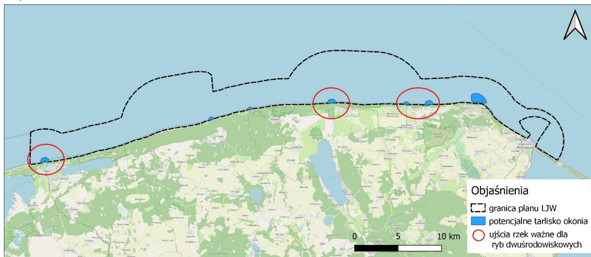
Ryc. 32. Miejsca cenne dla migracji ryb oraz potencjalne tarlisko okonia
