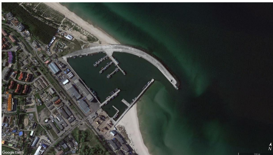
Ryc. 10. Falochrony osłaniające wejście do portu we Władysławowie.
