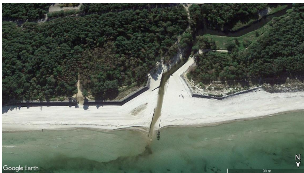
Ryc. 11. Zabudowa brzegu w rejonie ujścia Czarnej Wody.
