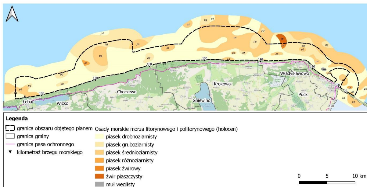
Ryc. 4. Osady morskie
