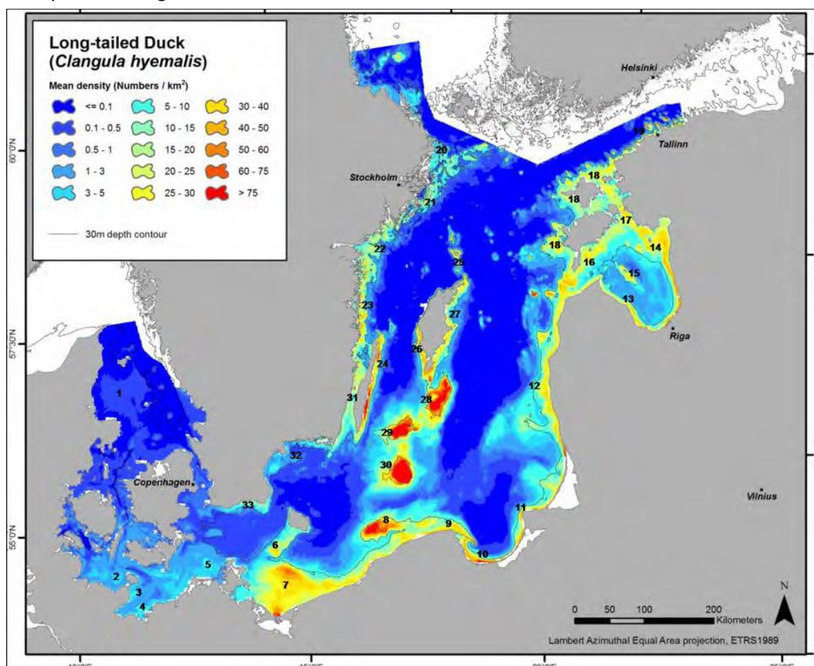
Ryc. 34. Rozmieszczenie i koncentracje zimowisk lodówki Clangula hyemalis na Morzu Bałtyckim w latach 2007-2009
