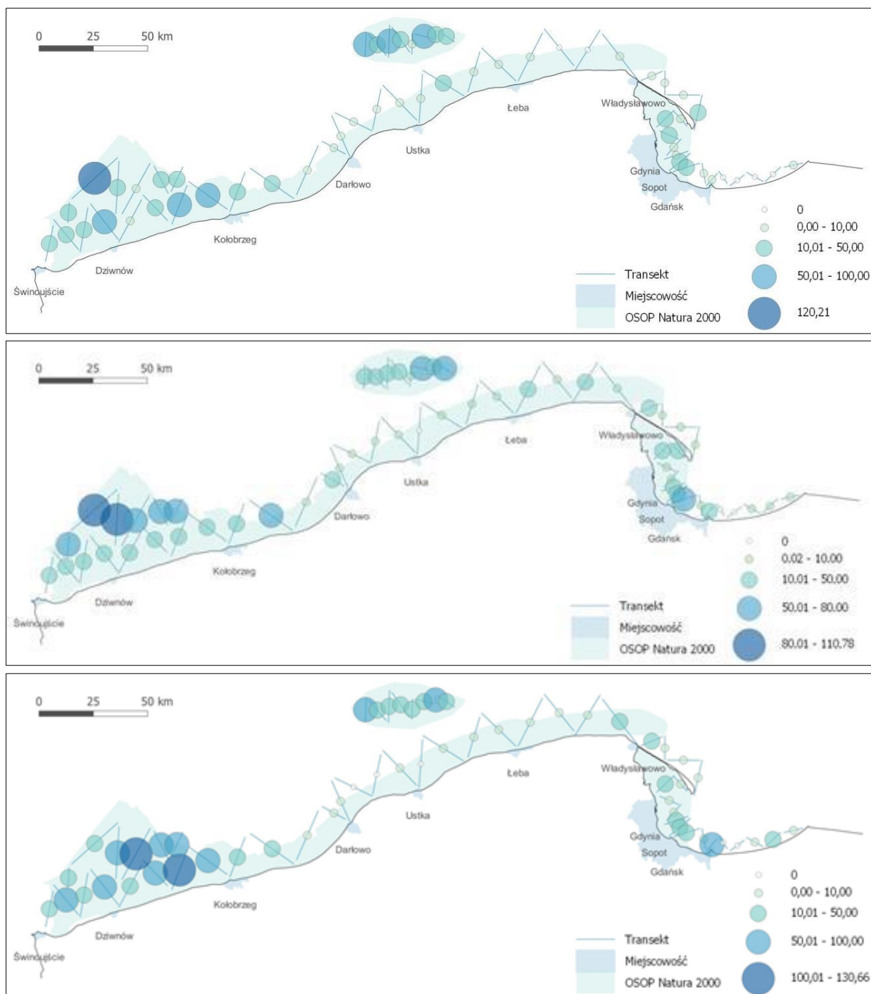
Ryc. 35. Wskaźniki zagęszczenia lodówki w polskiej strefie Bałtyku na podstawie wyników MZPM uzyskanych w 2019 (górze), 2020 (środek) i 2021 (dół) roku
