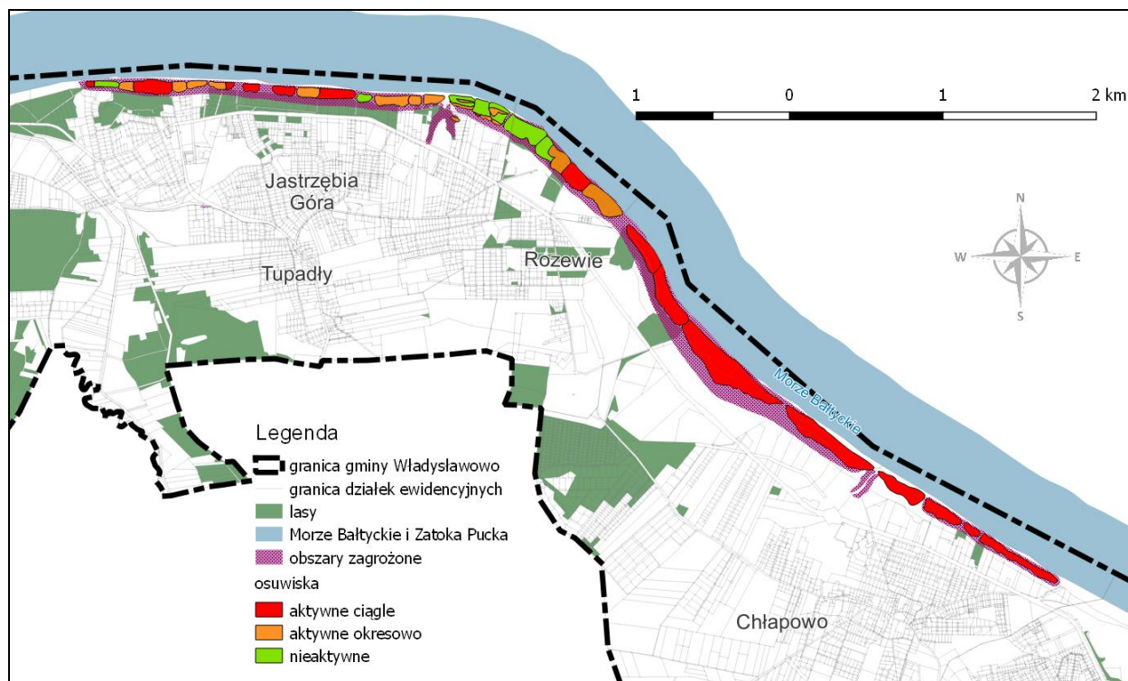
Ryc. 61. Obszary naturalnych zagrożeń geologicznych w rejonie klifów
