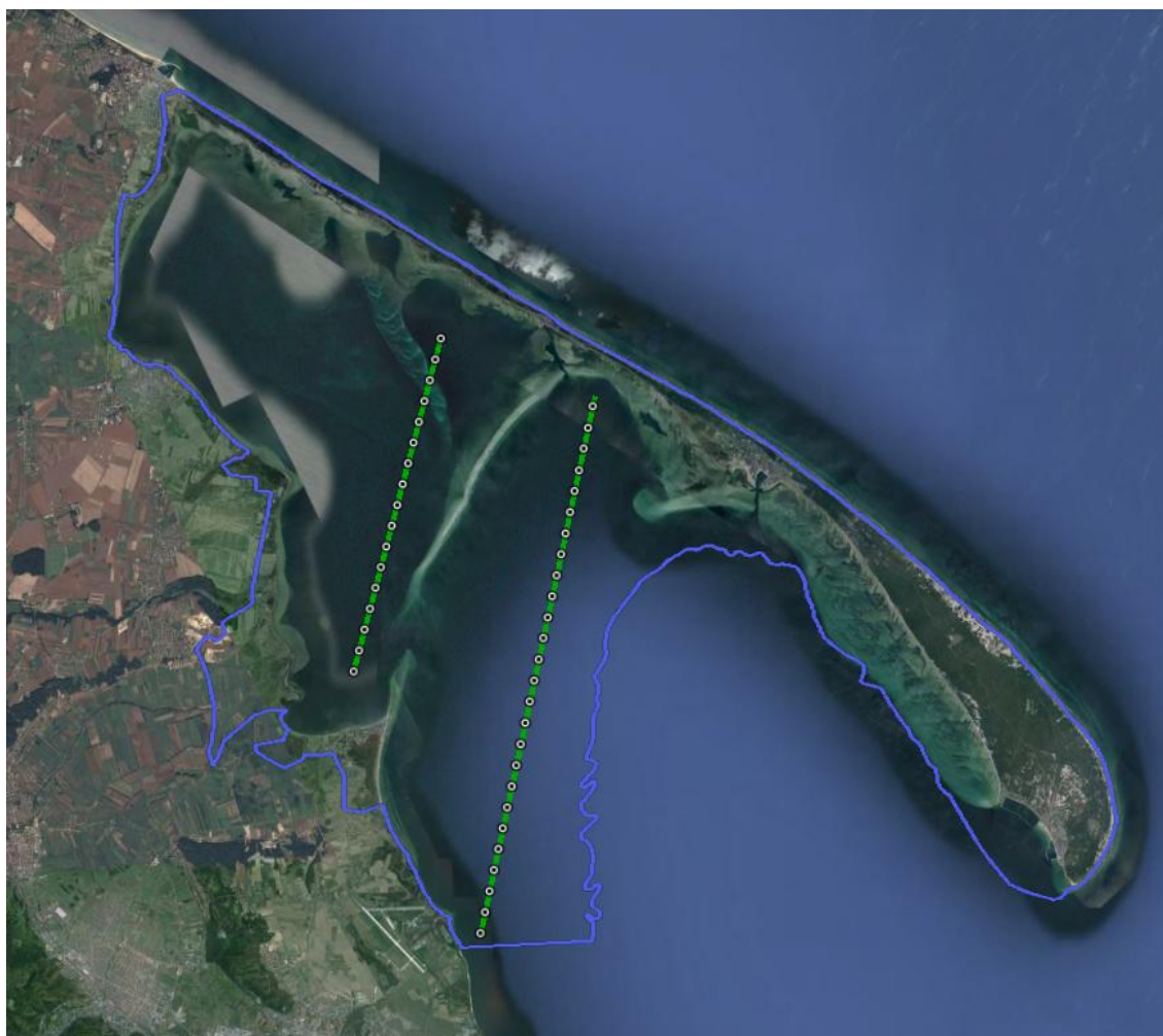
Rys. 1. Linie pomiarowe wzdłuż, których zostaną rozmieszczone C-POD-y
